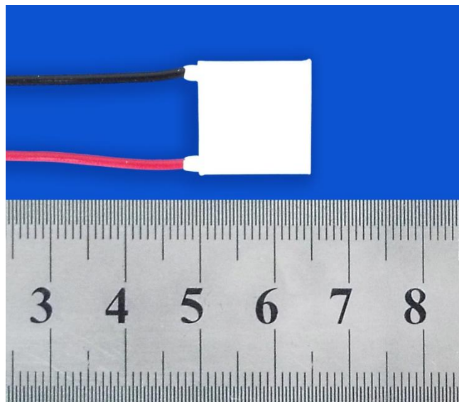
Figure 1. The Photo of Actual ATE1-TC-31-3AS
