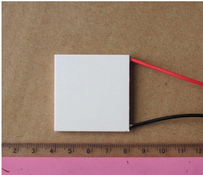
Figure 1. The Photo of Actual ATE1-241
