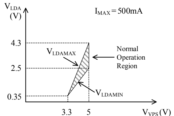
Figure 6. V_{VPS} & V_{LDA}
